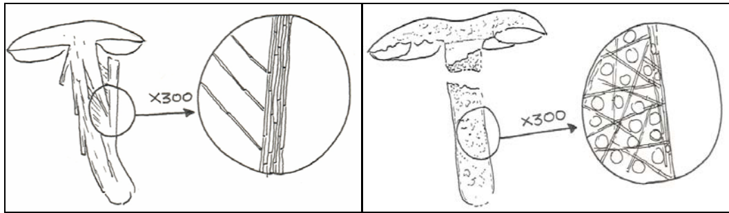
Fig. 6: Rotura fibrosa
